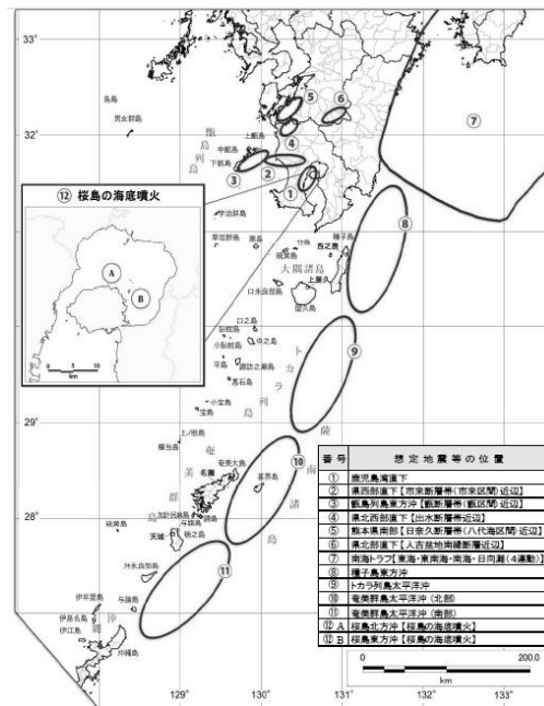
震源の位置
